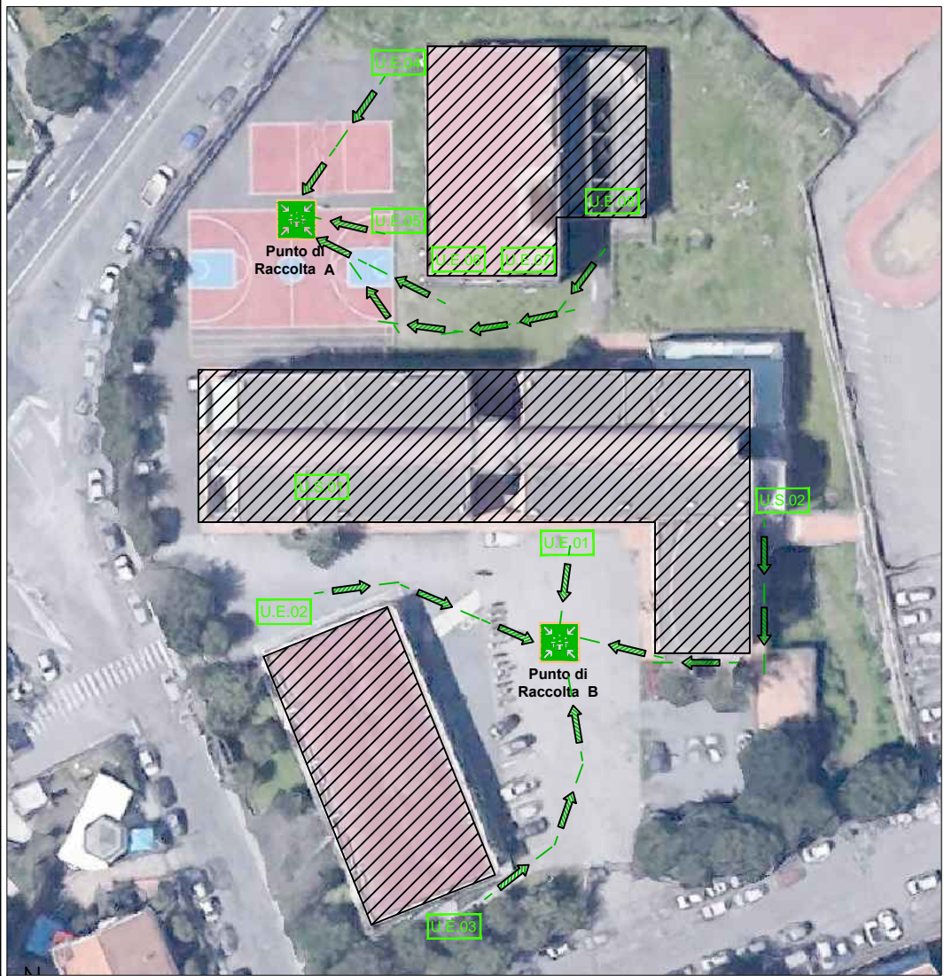
Stralcio Planimetrico
